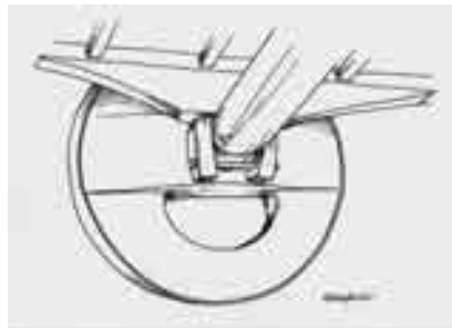
A “tuerca” suxeita as dúas treitoiras (debuxo de R. Marín, 2006)
